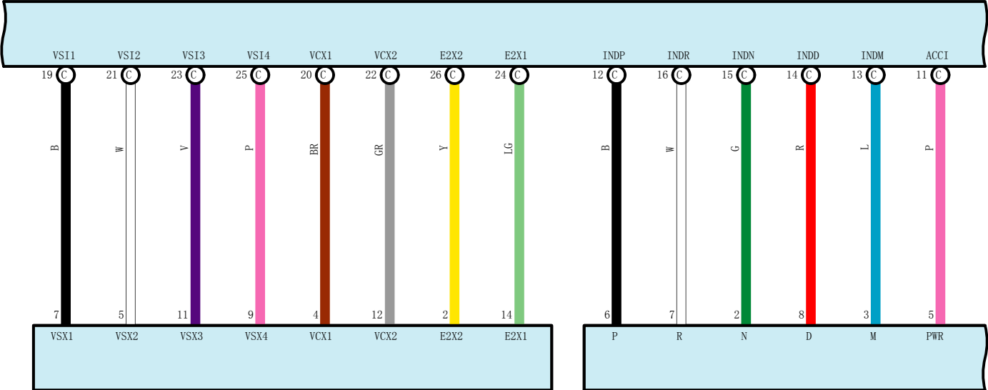
F175 换挡杆位置传感器 (换挡锁止控制单元总成)
